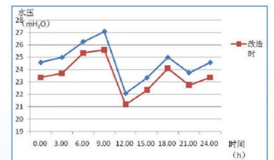
图2 最不利管段改造前、改造时压力变化
